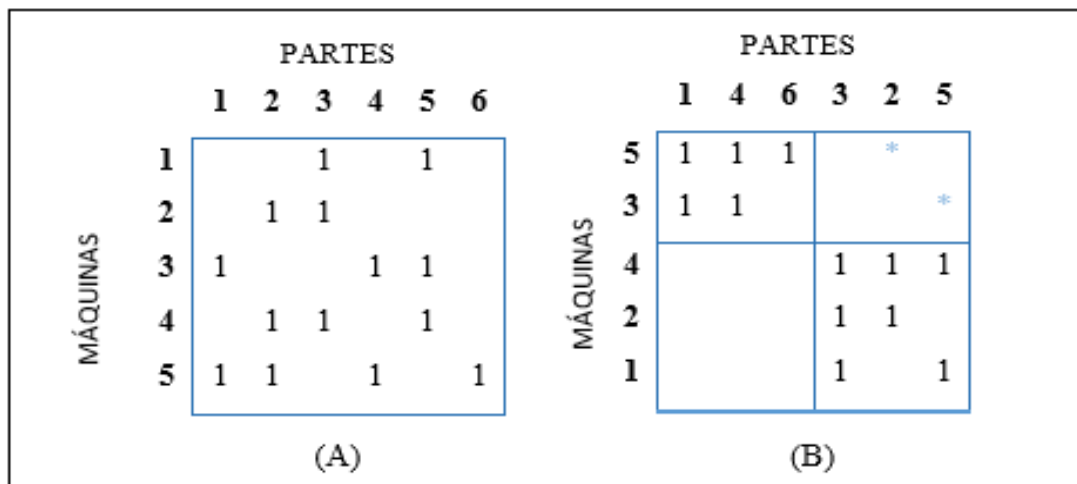
Figura 1 -Matriz de Incidência (A) Antes do agrupamento e (B) Após o agrupamento.
