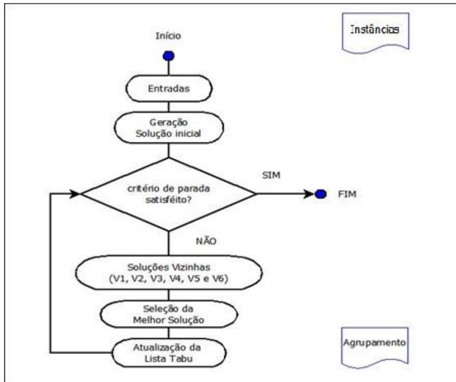
Figura 2- Arquitetura do Modelo BT proposto.
