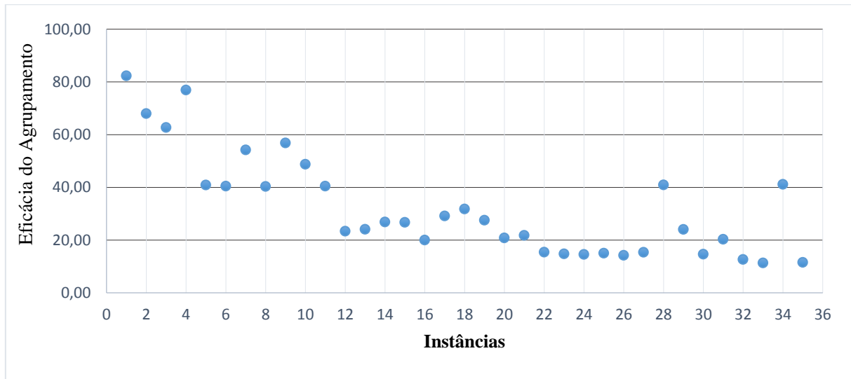
GRÁFICO 3 – Dispersão das soluções pela Eficácia do Agrupamento
