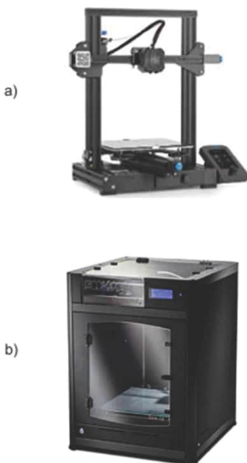
Figura 4 Modelos de impressoras 3D que operam com o processo fusão de filamento fundido do tipo (a) aberta e (b) fechada
