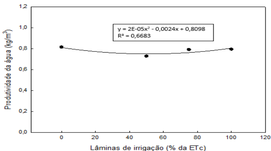
Figura 2 - Produtividade da água \text{kg m}^{-3} em função das lâminas de irrigação na cultura da soja.
