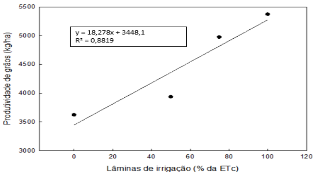
Figura 1 - Produtividade de grãos kg ha -1 em função das lâminas aplicadas
