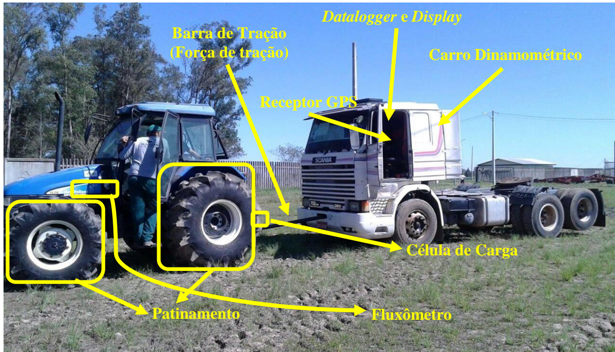
Figura 2 – Trator instrumentado e carro dinamométrico.
