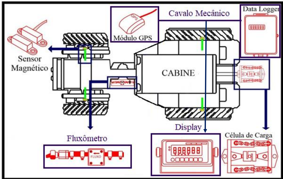
Figura 1 – Disposição dos sensores instalados no trator e sistema de aquisição de dados.
